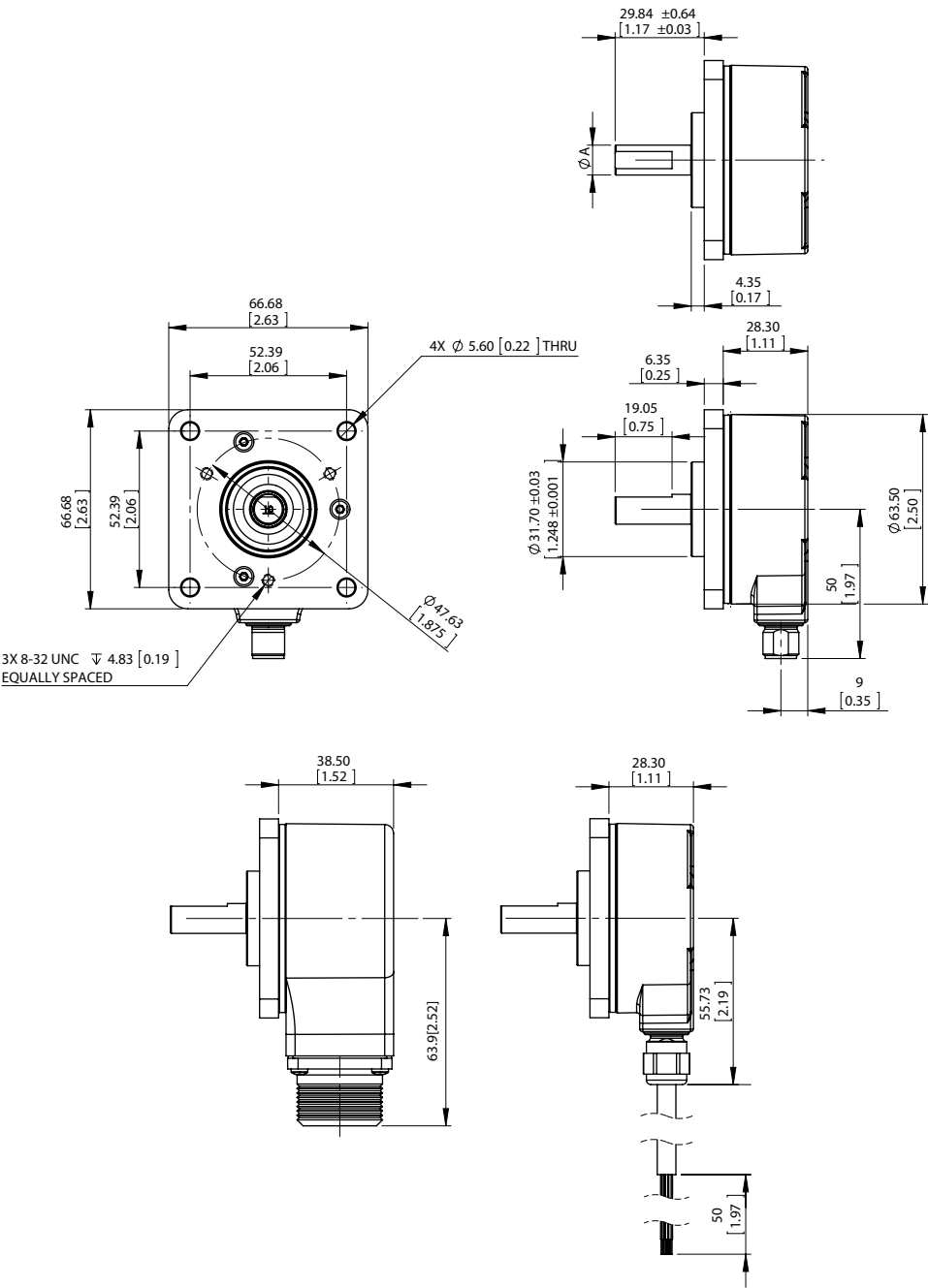
Plan coté DFS25, bride carrée, connecteur mâle radial de type M12 et MS, sortie de câble
