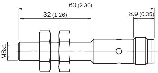
Dimensions en mm (inch)
