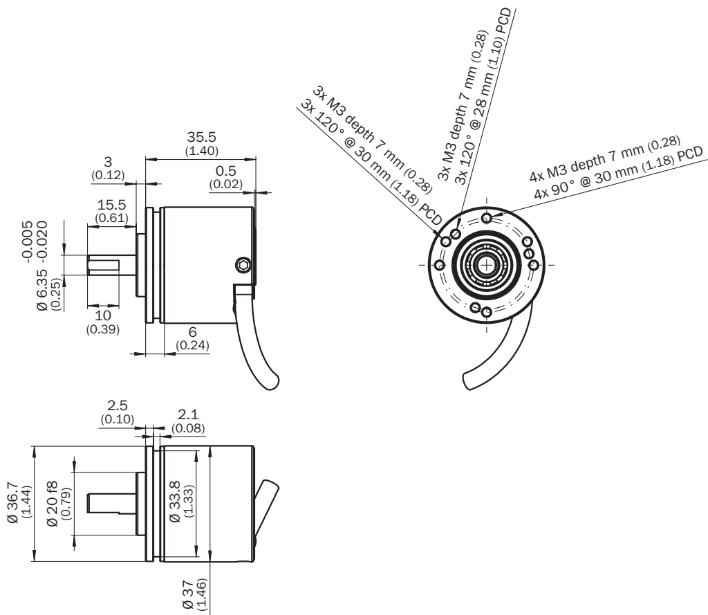
Dimensions en mm (inch)
