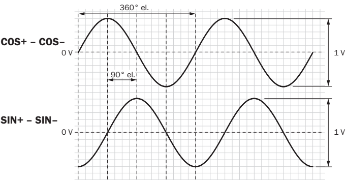
Diagrammes Signaux d'interface SIN COS selon la différence formée
