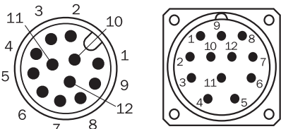
Vue connecteurs d'appareil M23 et M12 sur l'encodeur
