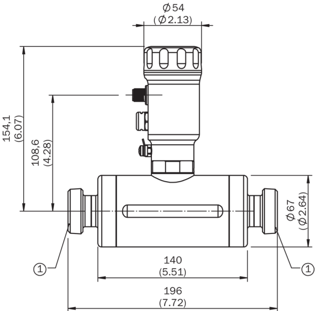
Dimensions en mm (inch)
