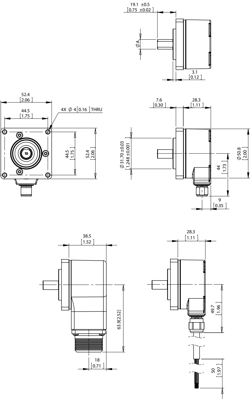
Plan coté DFS20, bride carrée, connecteur mâle radial de type M12 et MS, sortie de câble
