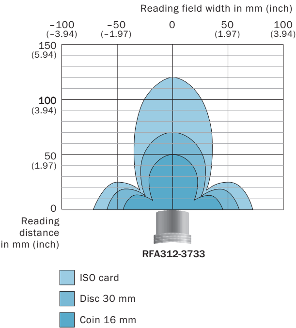
Diagramme des zones de lecture RFH630 Ethernet avec antenne externe
