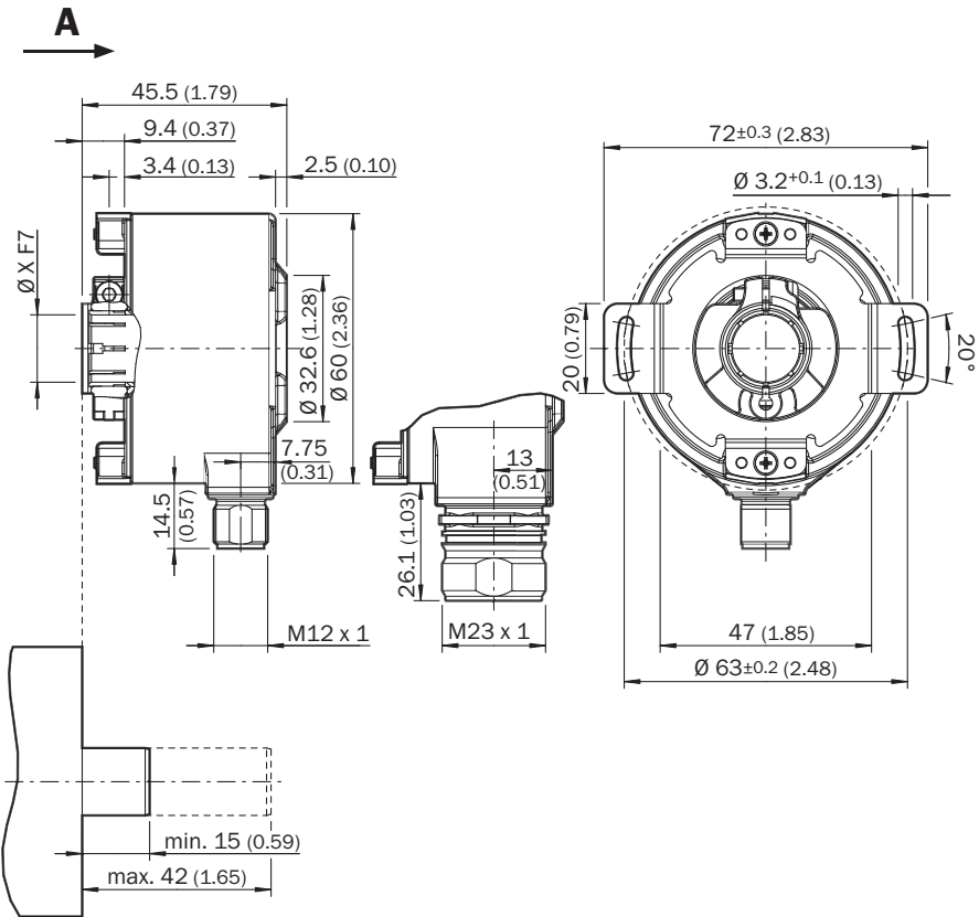
Plan coté Axe creux non traversant, connecteur mâle radial M12 et M23
