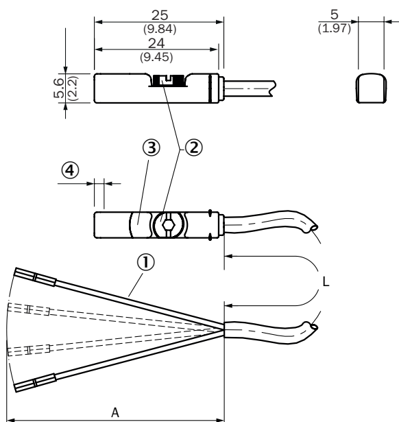
Plan coté Câble
