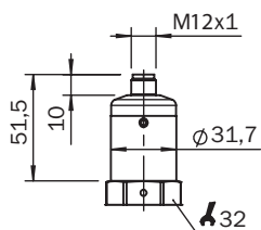
Maße in mm
