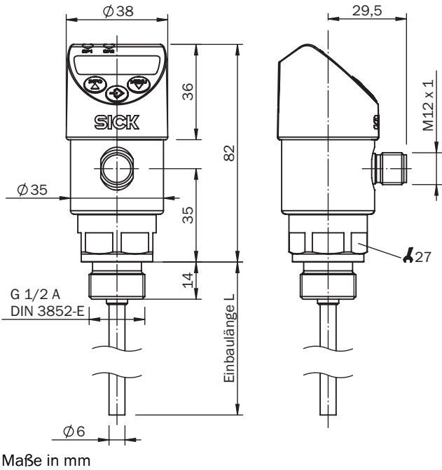
Maßzeichnung TBS mit Anschluss G \frac{1}{2} A nach DIN 3852-E
