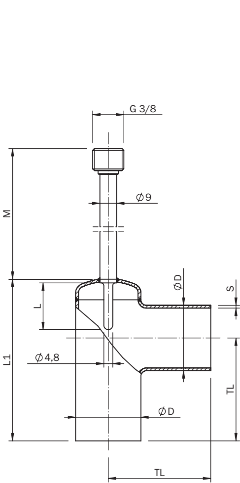
Schutzrohr mit Prozessanschluss
