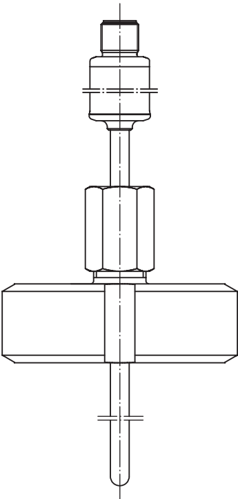
Gesamtdarstellung
