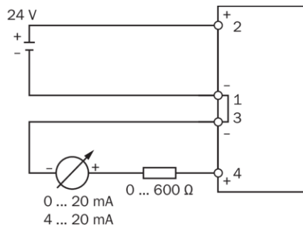
4 Leitertechnik
