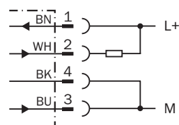
NPN-hellschaltend
