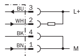
NPN-dunkelchaltend
