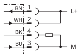
PNP-hellschaltend
