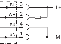
NPN-dunkelchaltend
