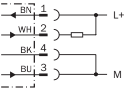
NPN-hellschaltend
