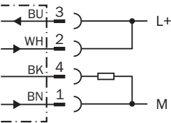
PNP-dunkelchaltend
