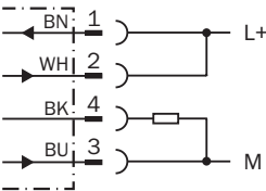
PNP-hellschaltend
