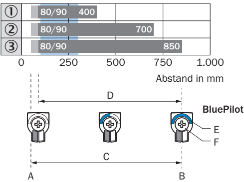
Empfohlener Schaltabstandsbereich für beste Performance
