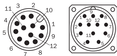
Ansicht Gerüststecker M23 und M12 am Encoder
