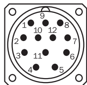
Ansicht Gerätestecker M23 an Leitung / Gehäuse
