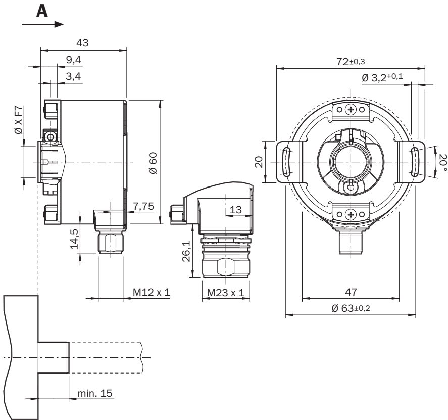
Maße in mm ① Leitungsdurchmesser = 5,6 mm +/- 0,2 mm Biegeradius = 30 mm
