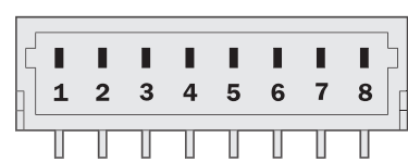
Anschlussart V
