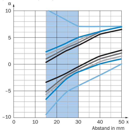
Transparente Glasscheibe vor Hintergrund (18 % Remission), Akzeptanzwinkel
