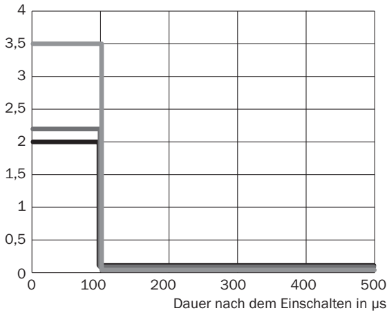
Typ. Stromaufnahme in A
