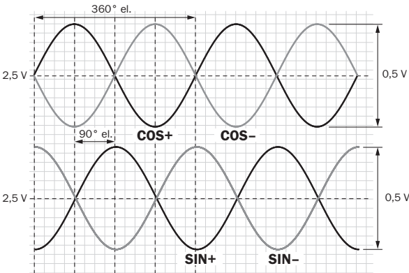
Diagramme Schnittstellensignale SIN/COS vor Differenzbildung
