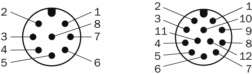
Ansicht Gerüstestecker M12 am Encoder
