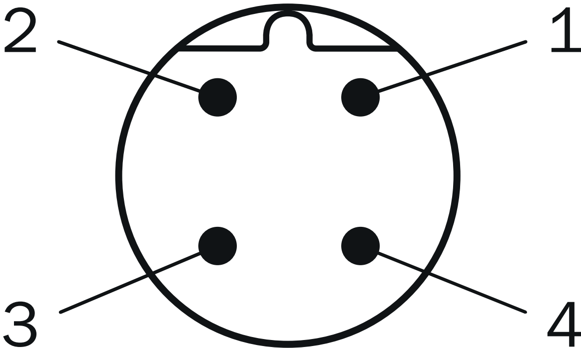
Versorgungsspannung
