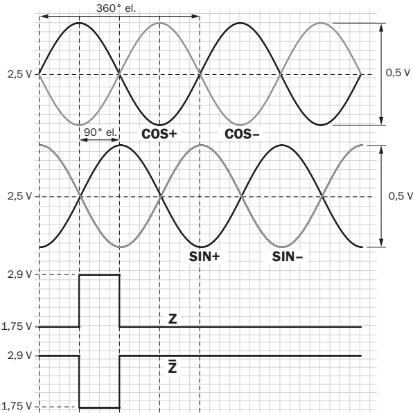
Diagramme Schnittstellensignale SIN/COS vor Differenzbildung
