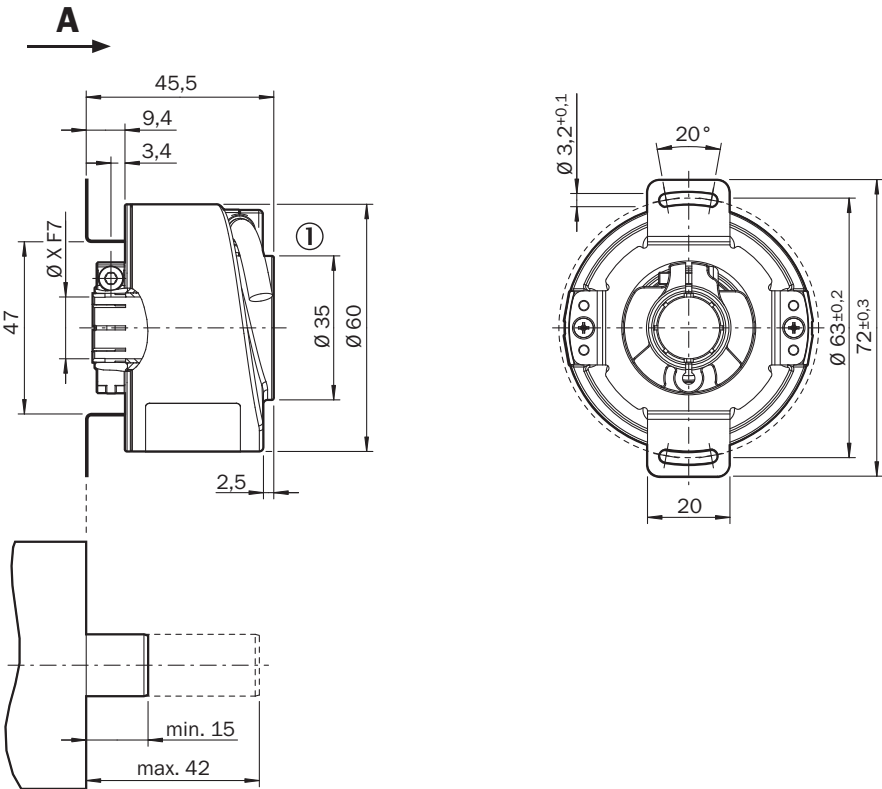
Maße in mm ① Leitungsdurchmesser = 5,6 mm +/- 0,2 mm Biegeradius = 30 mm
