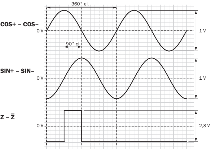
Diagramme Schnittstellensignale SIN/COS nach Differenzbildung
