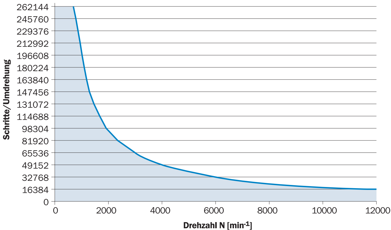
Drehzahlbetrachtung (n)
