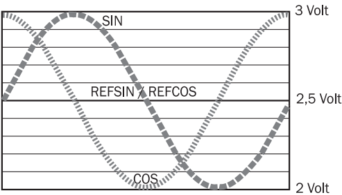
Diagramme Signalverlauf bei Drehen der Welle im Uhrzeigersinn mit Blick in Richtung "A" (siehe Maßzeichnung) 1 Periode = 360 ° : 1024
