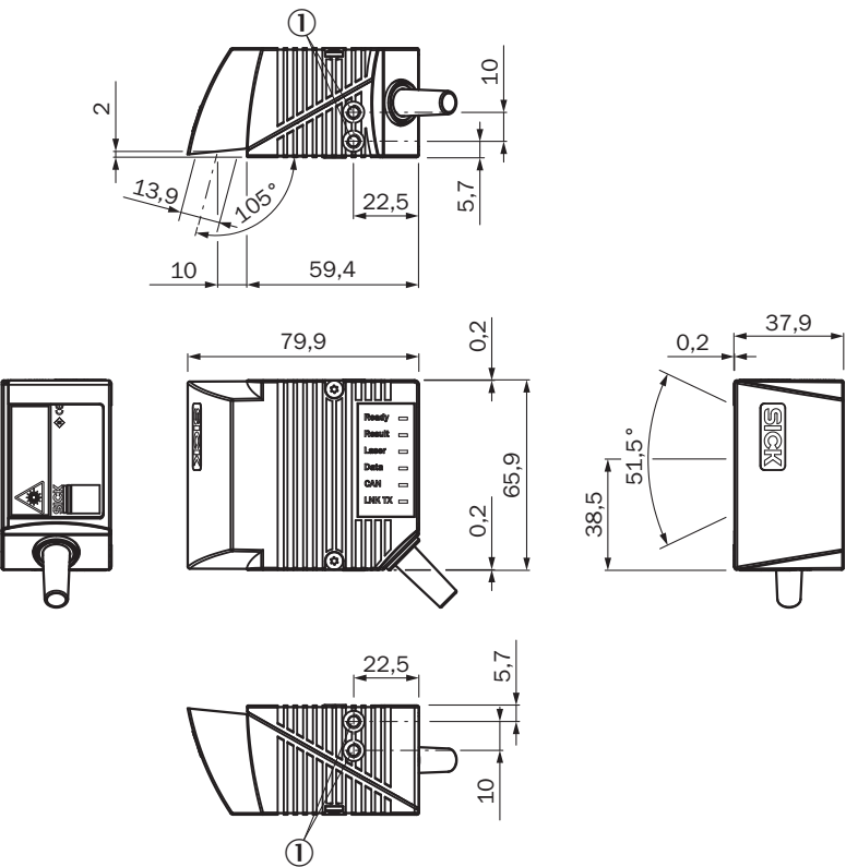
Maßzeichnung CLV62x Standard, seitlich
