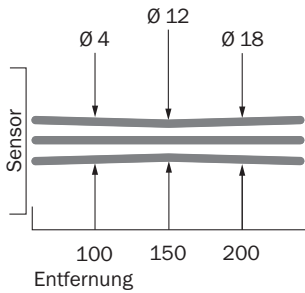
Tastweite 150 mm
